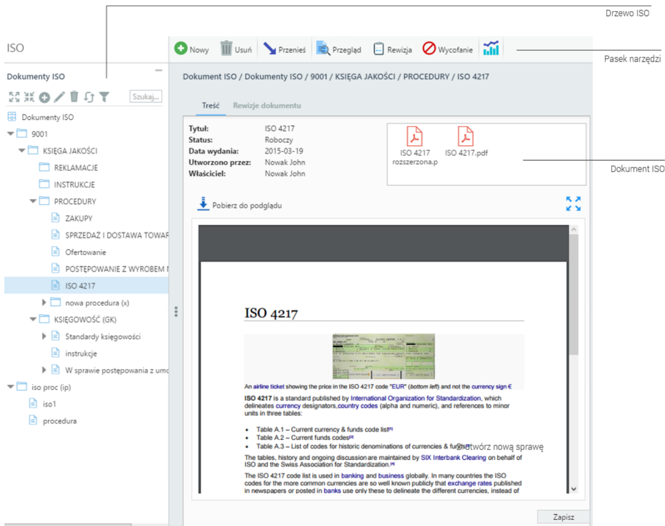
Ekran główny modułu ISO
