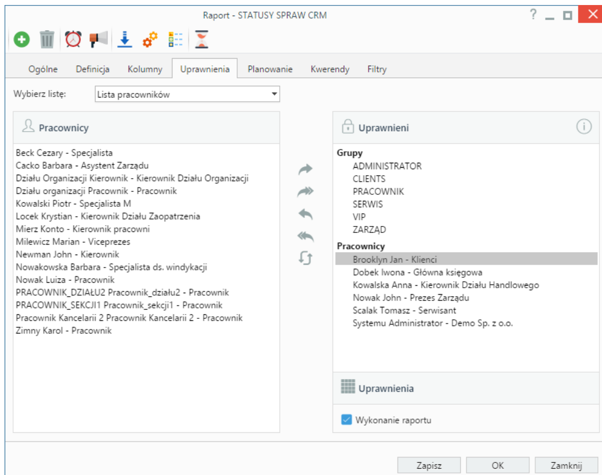
Okno edycji raportu - zakładka Uprawnienia
