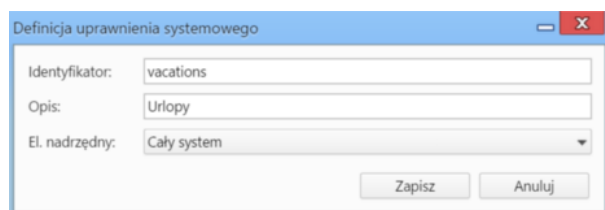
Okno definicji uprawnienia
